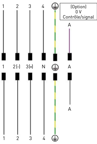
RETTBOX® ONE 32 A/400 V
